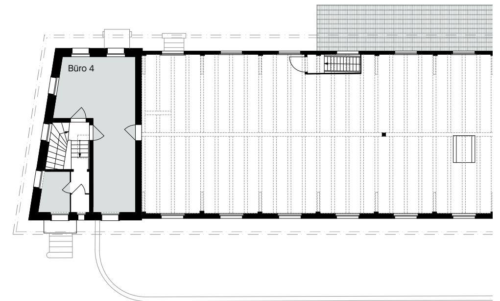
Grundriss 1. Obergeschoss, 1:200
