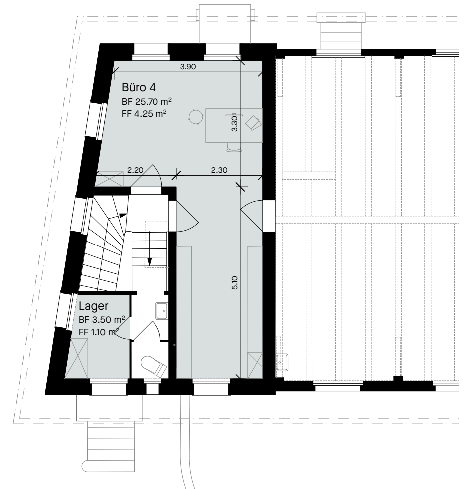
Grundriss 1. Obergeschoss, 1:100
