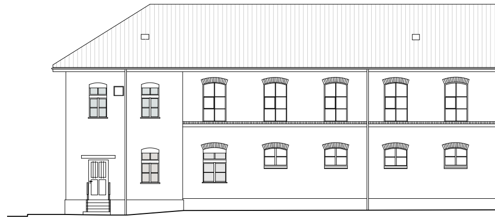
Ansicht Jägerstrasse, 1:200
