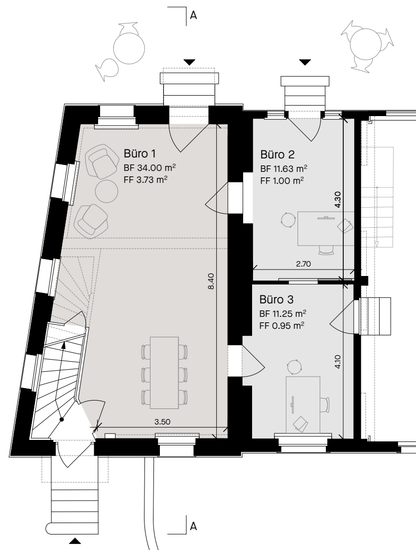
Grundriss Erdgeschoss, 1:100
