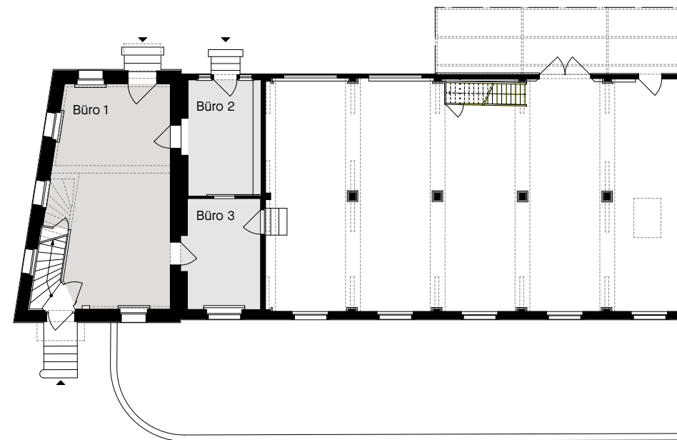
Grundriss Erdgeschoss, 1:200
